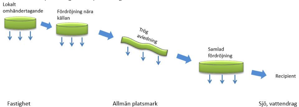
Bild 2: Schematisk bild för lokalt omhändertagande av dagvatten
